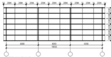
LSC-W8 Pfetten
