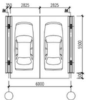
LSC-W6 Fundamente
